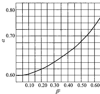
图 C. 2. 6-2 孔板流量系数图
